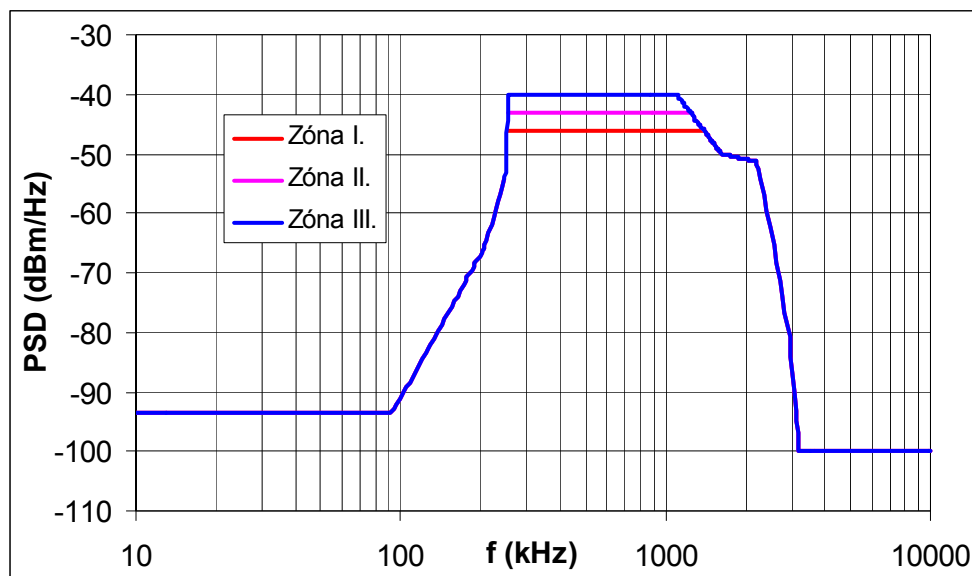
Obr. 5: Masky PSD-F pro sestupný provoz
